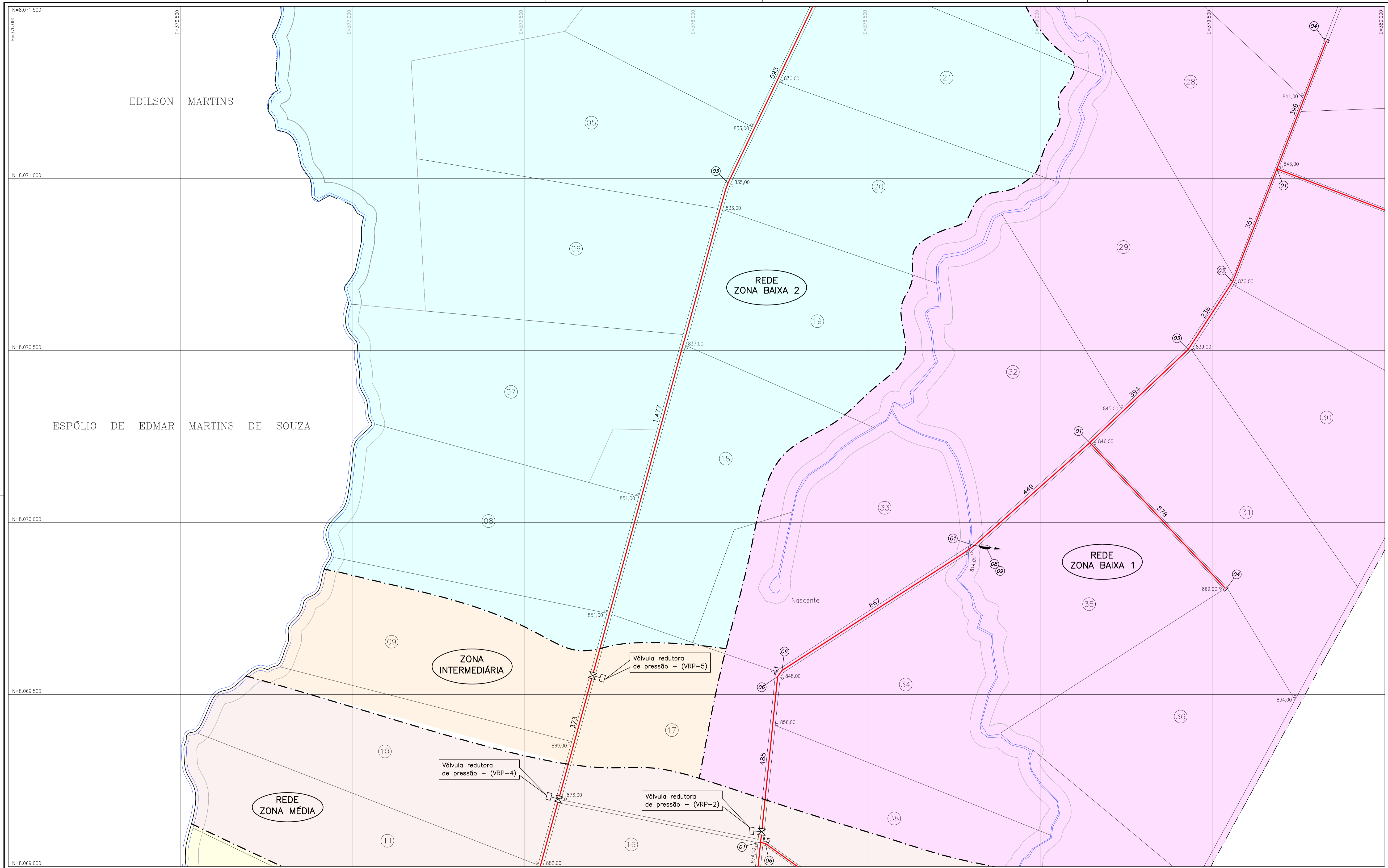
PLANTA - ESC.: 1:5000
